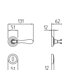
1421 maniglia per porta con rosetta door handle on rose
