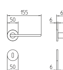
1751 maniglia per porta con rosetta door handle on rose
