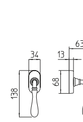
1422/DK martellina dk drehkipp system
