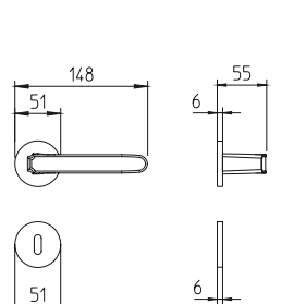
1871 maniglia per porta con rosetta door handle on rose
