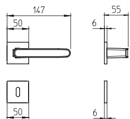
1871 maniglia per porta con rosetta door handle on rose
