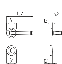
1341 maniglia per porta con rosetta door handle on rose
