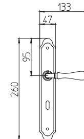
1420 con piastra door handle on backplate
