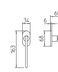
1752/DK martellina dk drehkipp system
