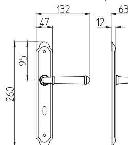
1340 con piastra door handle on backplate
