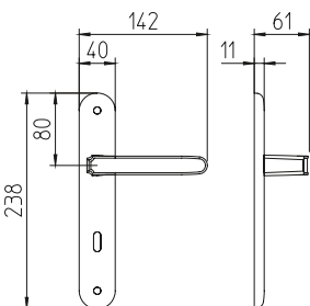
1870 con piastra door handle on backplate
