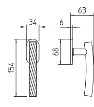
1732/DK martellina dk drehkipp system
