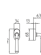
1342/DK martellina dk drehkipp system
