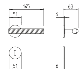
1731 maniglia per porta con rosetta door handle on rose
